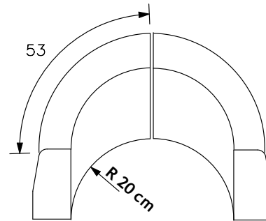
Curva a 90°
