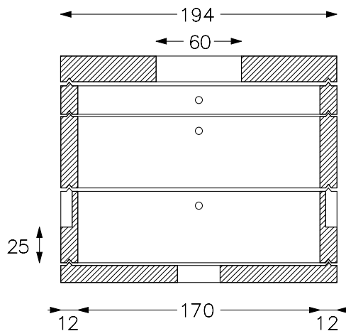
Sez. BB
