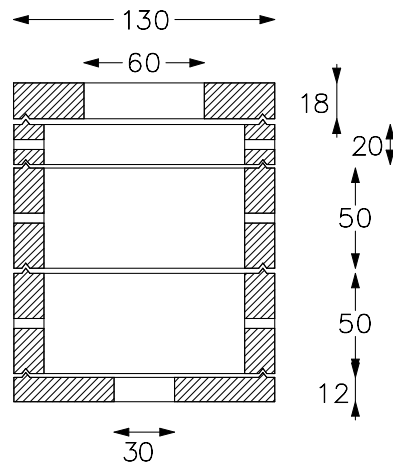
Sez. AA
